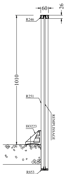
Version butant sous main courante
