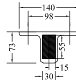
Sabot nez de dalle H0728 - H0738
