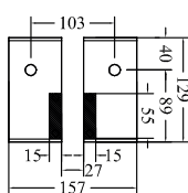
Sabot profilé H0252
