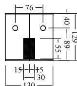
Sabot profilé H0252
