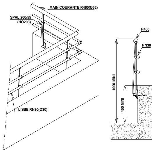
Triple lisses rondes sur barreau support moulé fixé contre muret.
