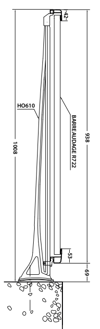
Version sur dalle butant sous main courante
