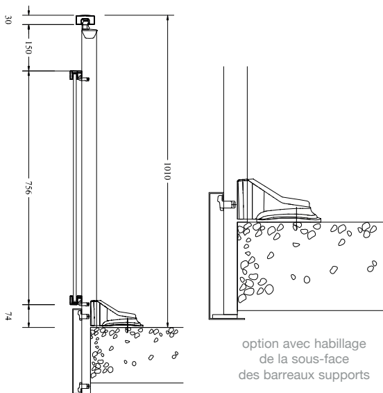
Principe d'habillage par fixation du bandeau filé R 819
