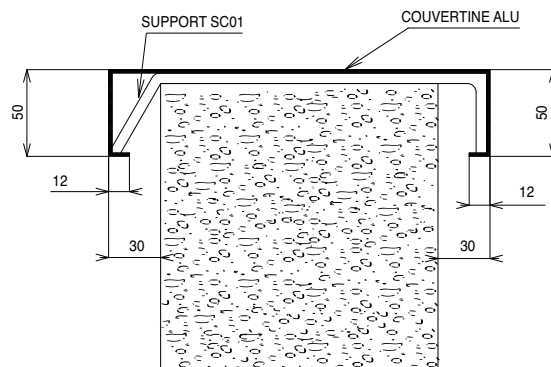
Détail couvertine
