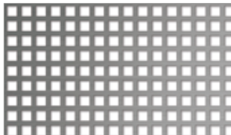
C6U9 44,44 % de vide
