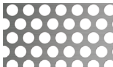
R15T21 46,28 % de vide
