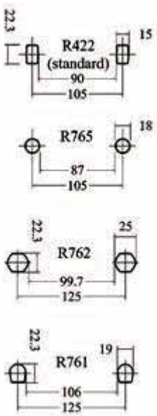
Détail du barreaudage
