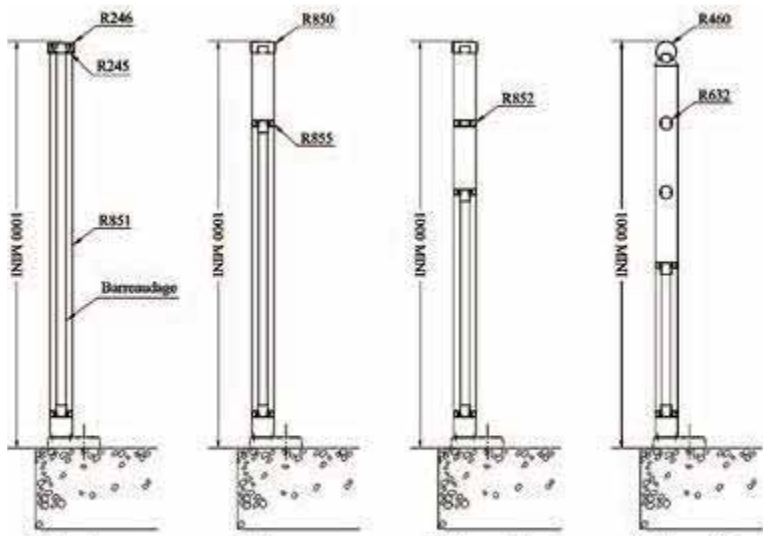
Butant Vide Vide + 1 lisse intermédiaire Vide + 2 lisses intermédiaires
