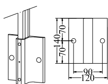
Détail embase HO949
