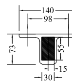
Sabot nez de dalle H0728 - H0738
