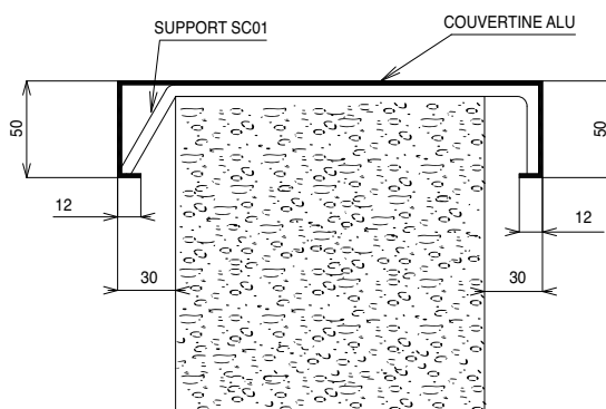
Détail couvertine
