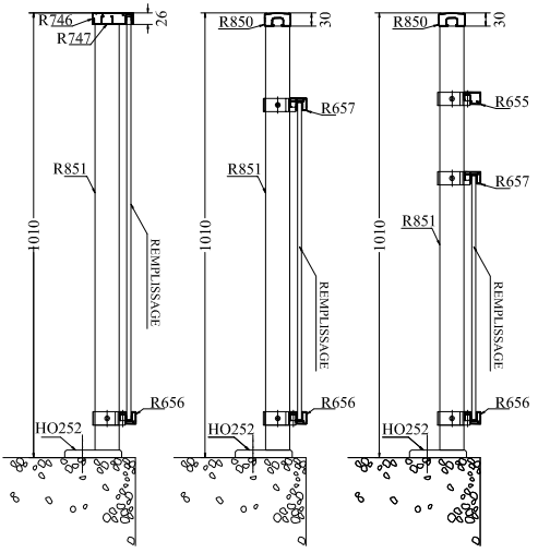
Butant Vide Vide + 1 lisse intermédiaire
