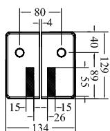
Sabot moulé H0723
