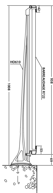
Version sur dalle butant sous main courante
