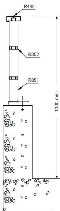
Version 2 lisses intermédiaires
