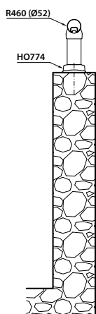
Version main courante seule sur potelet
