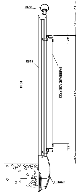
Version en nez de dalle vide sous main courante
