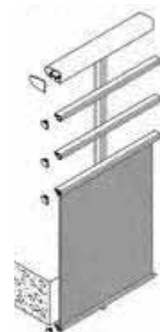
Version vide sous main courante avec lisses intermédiaires
