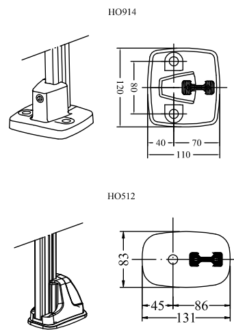
Sabots sur dalle
