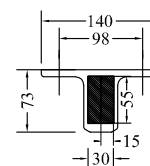
Sabot nez de dalle H0728 - H0738
