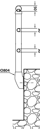
Version 3 lisses fixées à l'anglaise
