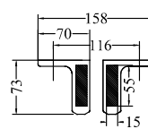
Sabot nez de dalle H0728 - H0738
