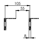
Détail de barreaudage R336
