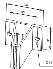
Sabot de fixation HO904
