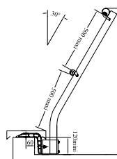
Modèle incliné Fixation à 30°
