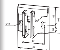
Sabot de fixation HO600
