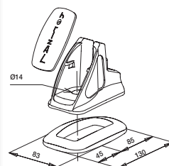
Sabot de fixation HO612 ou HO512
