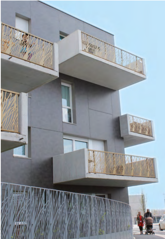
AREAL butant sous main courante remplissage en tôle découpée laser.
