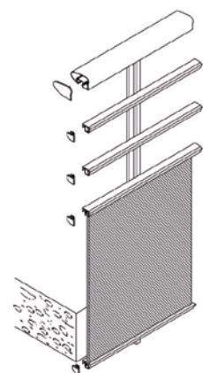
Version vide sous main courante avec lisses intermédiaires
