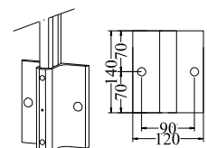
Détail embase HO949
