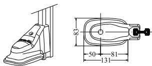
Détail embase HO419
