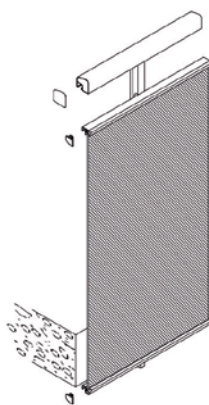
Version vide sous main courante
