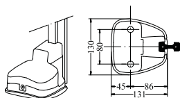
Détail embase HO872
